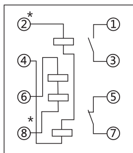
DT-1接线图
